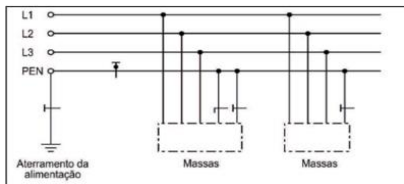
Figura 4- Esquema TT
