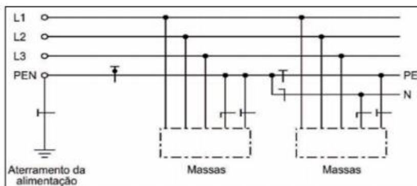
Figura 2- Esquema TN-C-S
