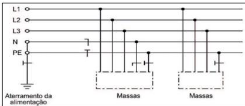
Figura 1 — Esquemas TN-S
